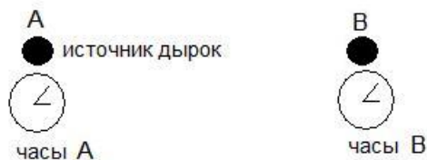
Рис.6 Схема обнаружения вакуумных дырок (Декартовой пустоты) при помощи прецизионных атомных часов.
