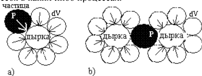
Рис. 3 Взаимодействие вакуумных дырок с веществом. Частица P, вместе с квантами пространства-времени dV образует Декартов сосуд вокруг дырки.
